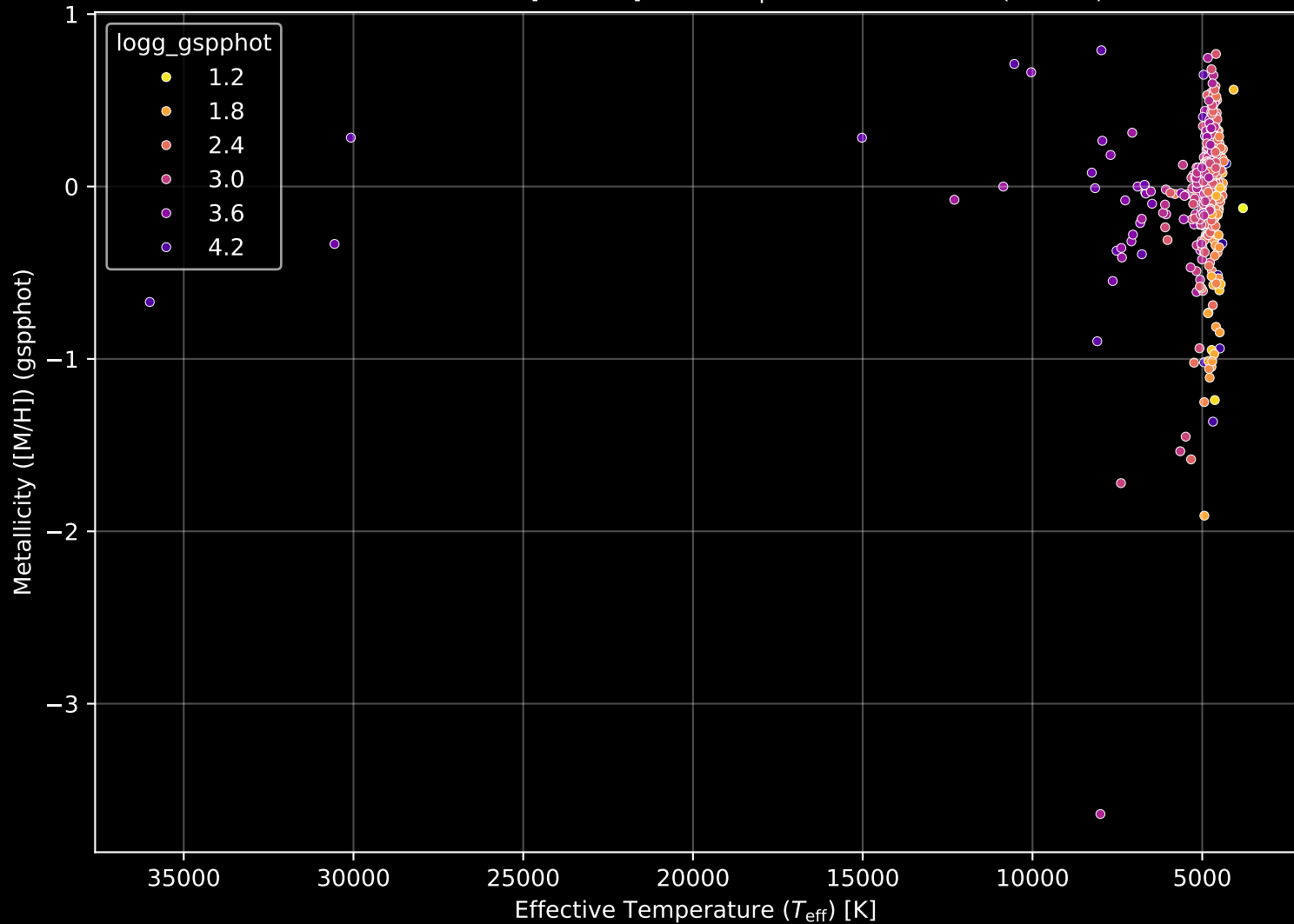
APOGEE DR17 Field: [330+04] Stellar Population Parameters (n= 577)
